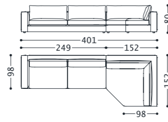
01LAGC10 (1LAGD3SX + 1LAGTRSP) 02LAGC10 (2LAGD3SX + 2LAGTRSP)
