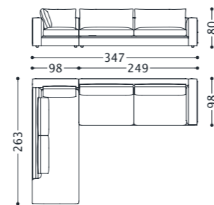
01LAGC9 (1LAGMERSX + 1LAGD3DX) 02LAGC9 (2LAGMERSX + 2LAGD3DX)
